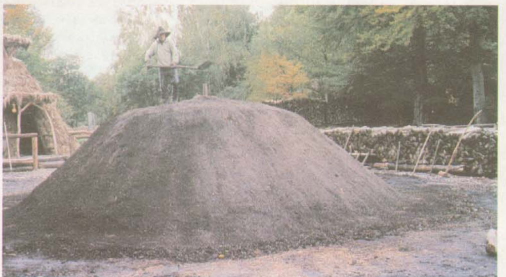
Anzündung des Meilers in der Köhlerei Stemberghaus.
